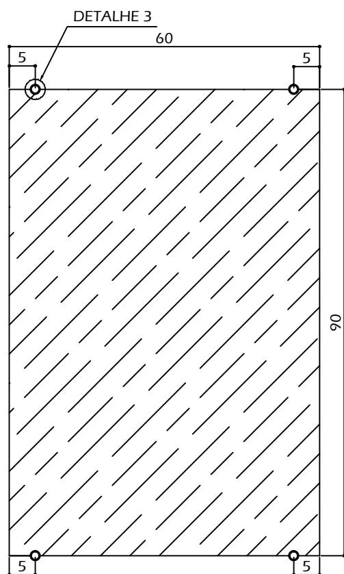
ESPELHO 90X60 COM PARAFUSO FINESSON
