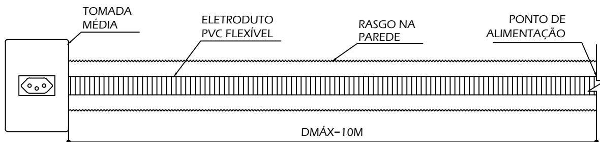
TIPO 5 - TOMADA 2PT - 10A - 250V
