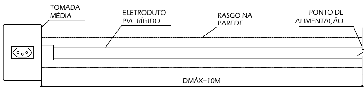
TIPO 4 - TOMADA 2PT - 10A - 250V
