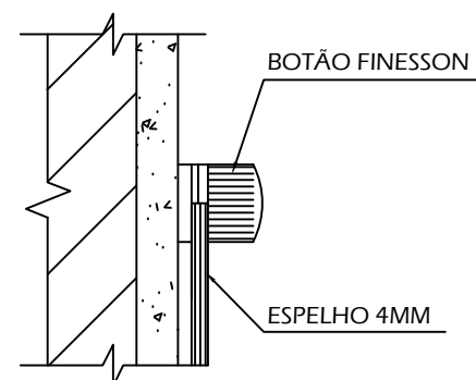
DETALHE 3
