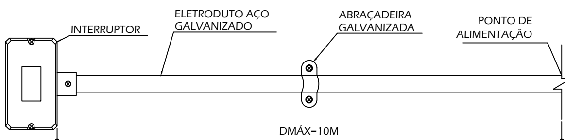
TIPO 2 - INTERRUPTOR SIMPLES DE SOBREPOR
