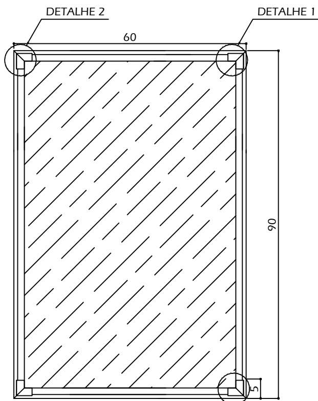
ESPELHO 60X90 COM MOLDURA EM ALUMÍNIO
